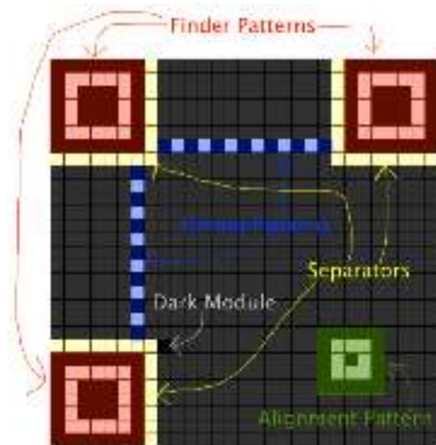
Gambar 2.2. Pola QR-Code (Xu, 2015)
