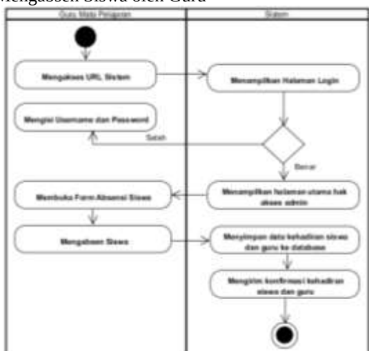
Gambar 3.8. Activity Diagram mengabsen siswa 7). Mencetak kehadiran siswa oleh wali kelas
