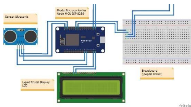
Gambar 3. Rancangan rangkaian perangkat keras
