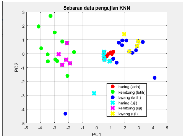
Gambar 5. Sebaran Data Pengujian
