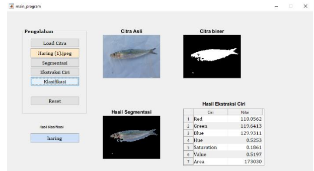
Gambar 6. Running System Klasifikasi
