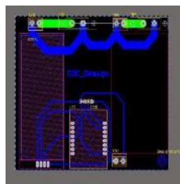
Gambar 3 Wiring Perangkat PCB dan Mikrokontroler.
