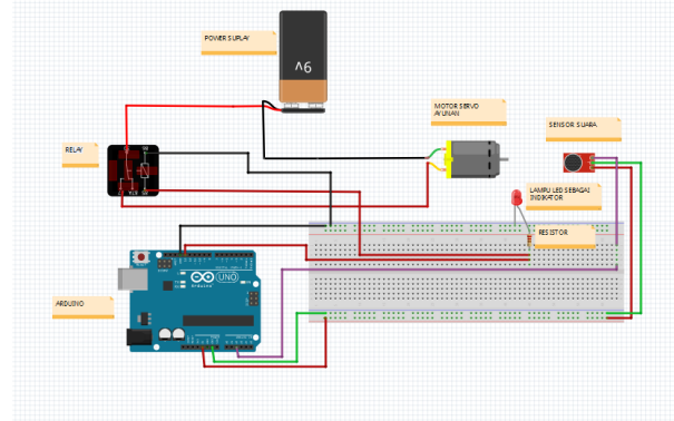
Gambar 2. Pra Rancangan Ayunan Bayi
