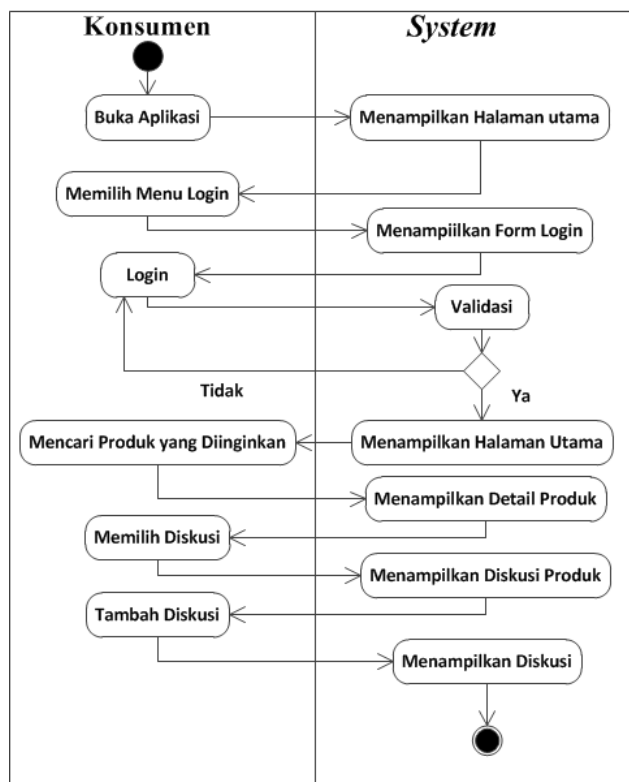
Gambar 8. Activity Diagram Diskusi Produk
