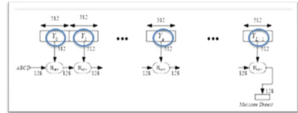
Gambar 7. Pengolahan Pesan Dalam Blok 512 Bit
